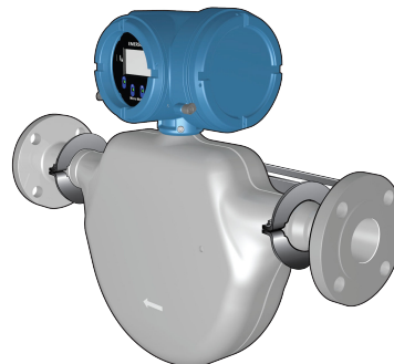
Figura 3-11: CMFS025, CMFS040 o CMFS050 montado en pared usando el soporte
