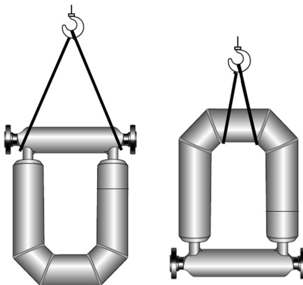
Figura 3-1: Puntos de elevación aceptables
